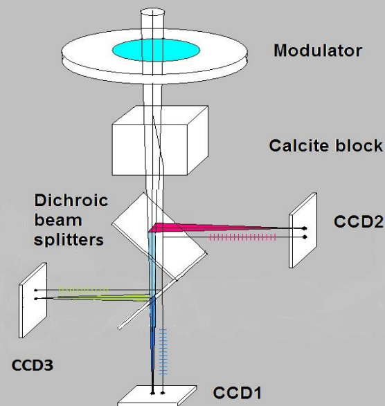
DIPOL-2 polarimeter
