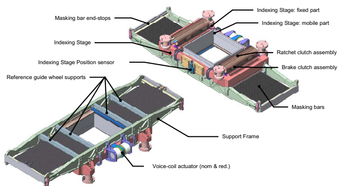
図 2.10: CSU の機構図。
