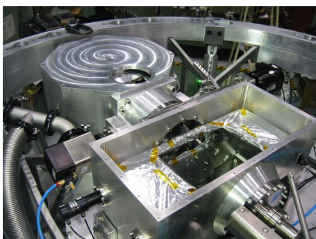
図 2.9: 左 : MOIRCS の MOS スリット交換機構の実物。
